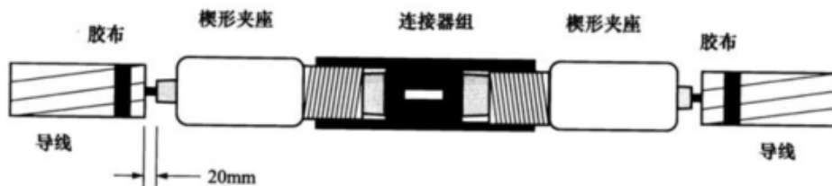
图 B.6 楔接式接续管安装位置
