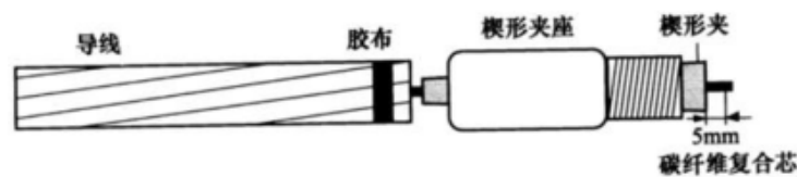
图 C.4 碳纤维复合芯穿入楔形夹座、楔形夹
