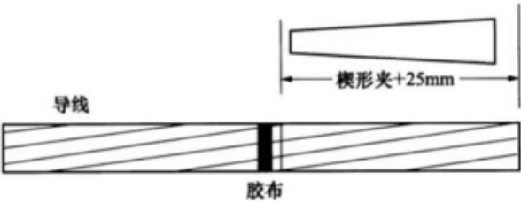
图 B.2 画印记
