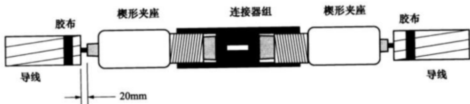
图 C.6 楔接式接续管安装
